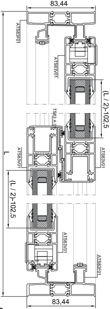
B-B ÖLÇEK / Scale: 1/2
