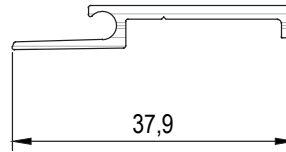
02.03.24 (PVC Profil)
