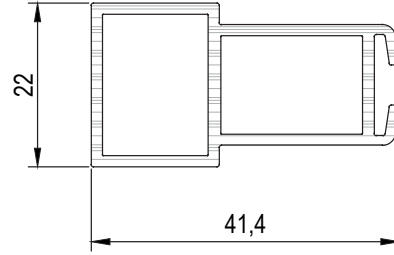
02.03.23 (PVC Profil)
